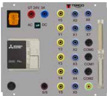
TF8050-FX3s PLC-modul Mitsubishi Melsec FX3s 6 ingångar, 8 utgångar Ström max för applikation: 24V, 3A
